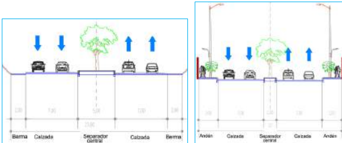
FIGURA 94. SECCIÓN TRANSVERSAL TIPO 9 Y 10 - PMMM 2011-2030
