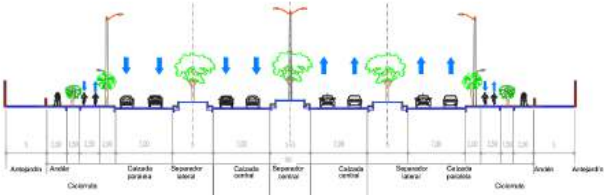
FIGURA 89. SECCIÓN TRANSVERSAL TIPO 2 - PMMM 2011-2030
