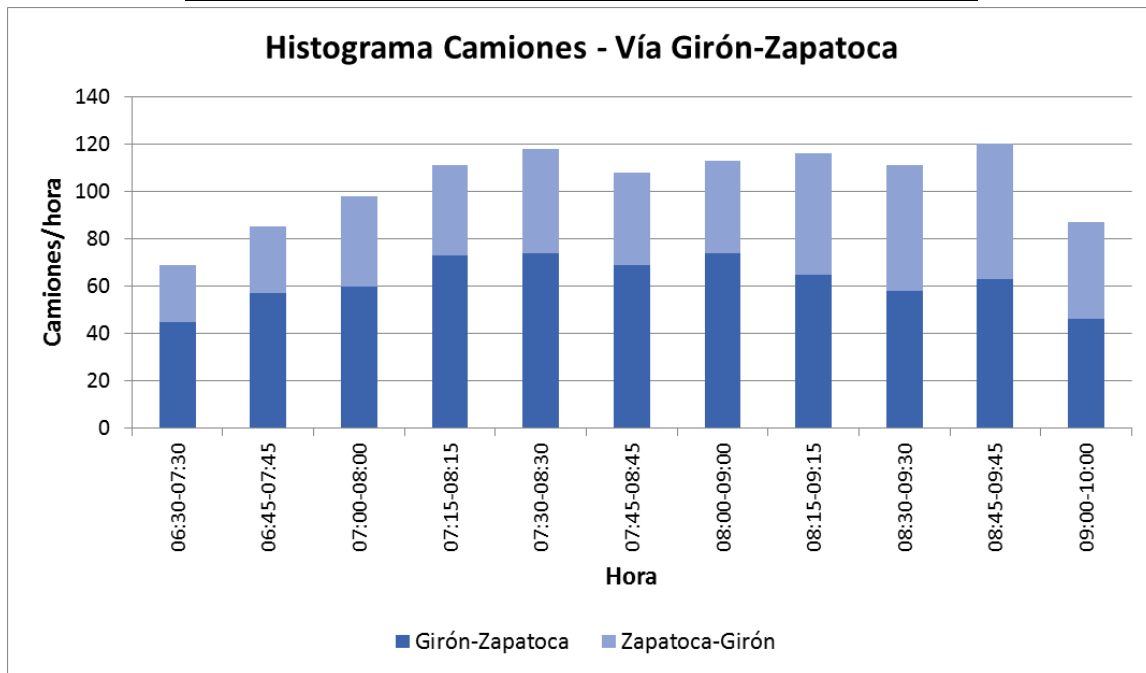
FIGURA 161. VOLÚMENES DE CAMIONES EN LA VÍA GIRÓN – ZAPATOCA
