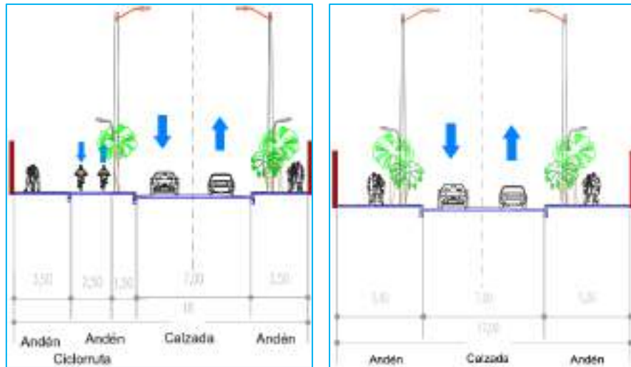
FIGURA 95. SECCIÓN TRANSVERSAL TIPO 11 Y 12 - PMMM 2011-2030
