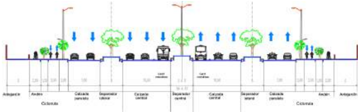
FIGURA 88. SECCIÓN TRANSVERSAL TIPO 1 - PMMM 2011-2030
