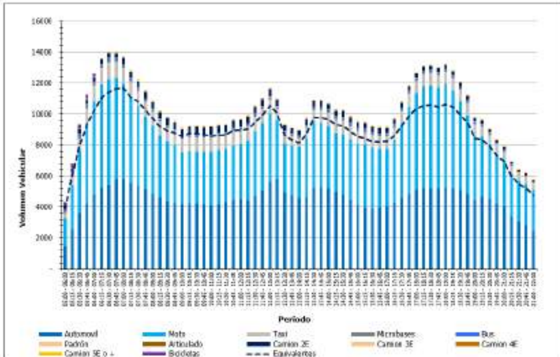
FIGURA 130. ESTACIÓN MAESTRA AV. FLORIDABLANCA/ANILLO VIAL
