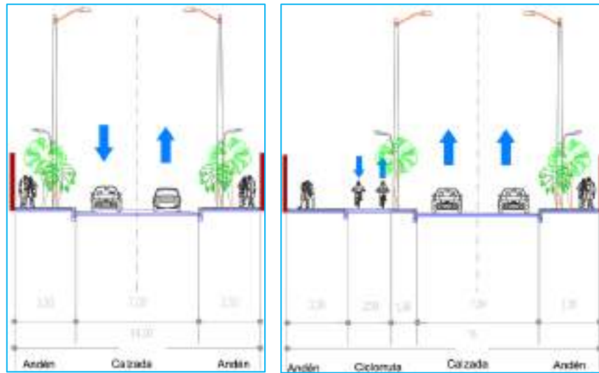
FIGURA 96. SECCIÓN TRANSVERSAL TIPO 13 Y 14 - PMMM 2011-2030
