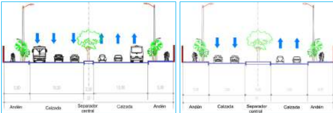
FIGURA 92. SECCIÓN TRANSVERSAL TIPO 5 Y 6 - PMMM 2011-2030
