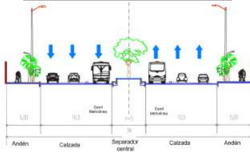
FIGURA 91. SECCIÓN TRANSVERSAL TIPO 4 - PMMM 2011-2030
