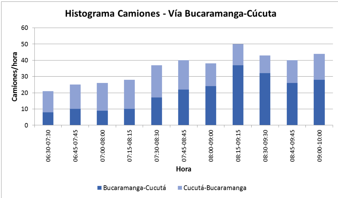
FIGURA 160. VOLÚMENES DE CAMIONES EN LA VÍA BUCARAMANGA – CÚCUTA
