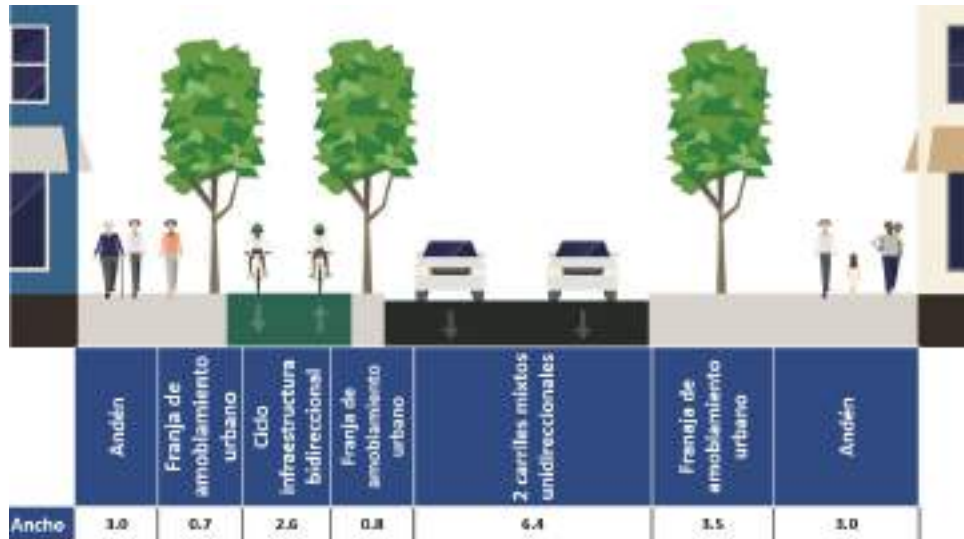
FIGURA 100. SECCIÓN TRANSVERSAL TÍPICA TIPO A EN EL TRAMO DE UIS-PARQUE DE LOS NIÑOS.
