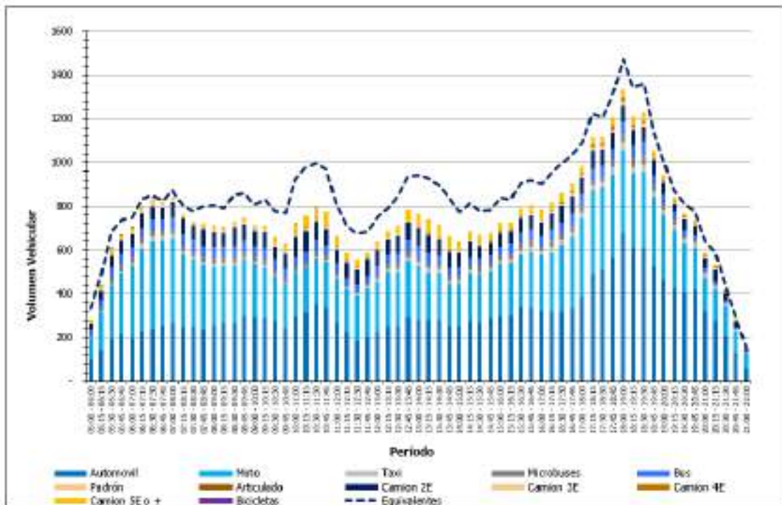
FIGURA 132. ESTACIÓN MAESTRA VIJAGUAL
