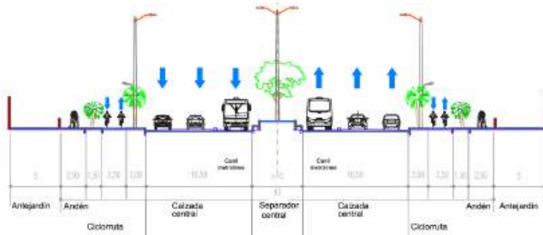
FIGURA 90. SECCIÓN TRANSVERSAL TIPO 3 - PMMM 2011-2030
