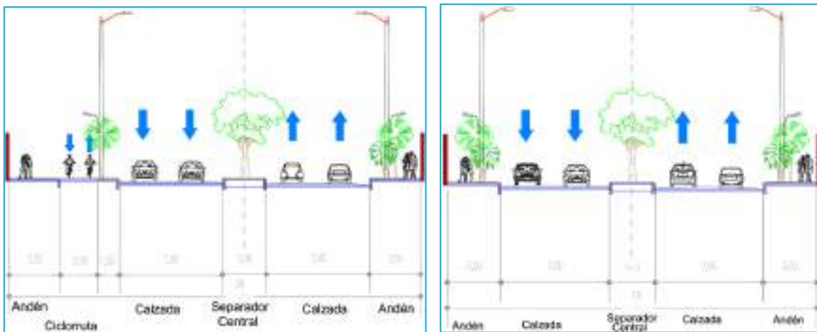
FIGURA 93. SECCIÓN TRANSVERSAL TIPO 7 Y 8 - PMMM 2011-2030
