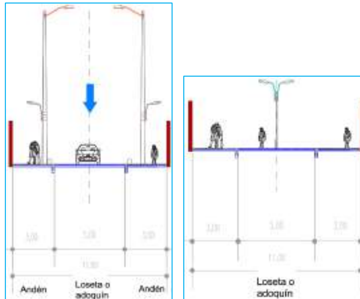
FIGURA 98. SECCIÓN TRANSVERSAL TIPO 17 Y 18 - PMMM 2011-2030
