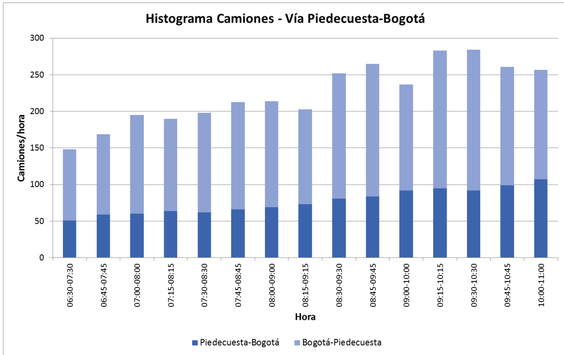
FIGURA 162. VOLÚMENES DE CAMIONES EN LA VÍA PIEDECUESTA – BOGOTÁ
