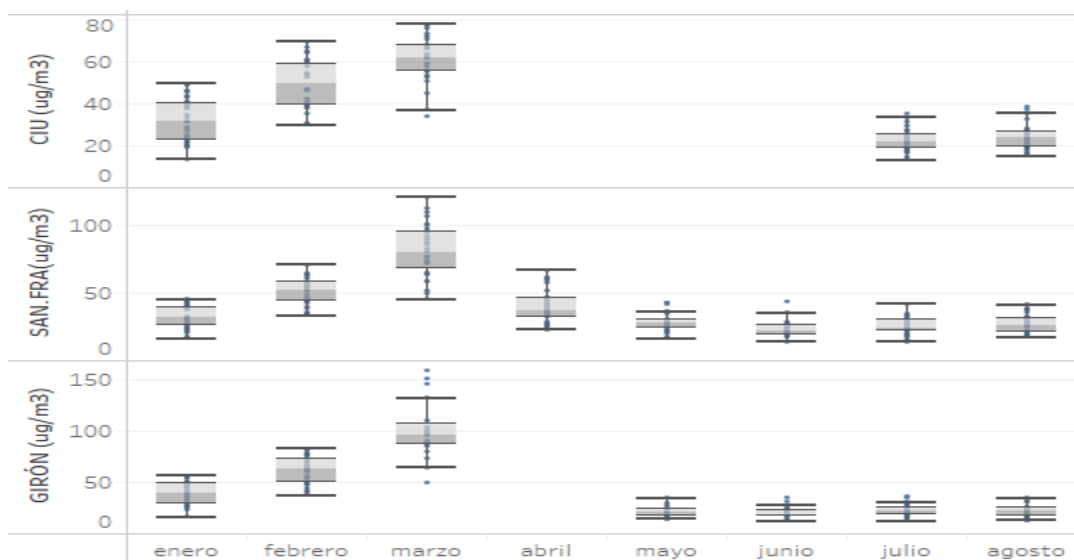
Figura 4 Diagrama de cajas mensual PM_{10}
