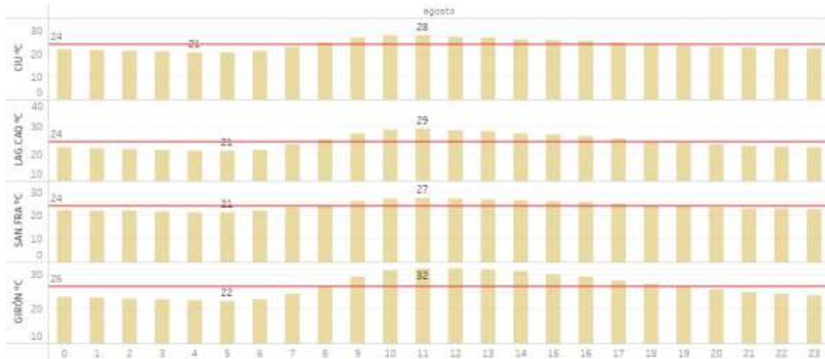
Figura 10 Comportamiento horario de la temperatura °C
