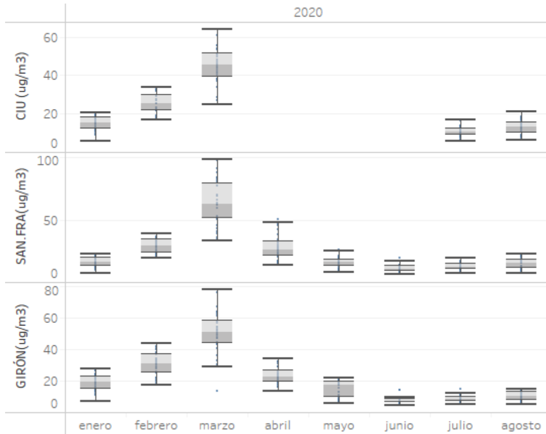
Figura 7 Diagrama de cajas PM_{2.5}
