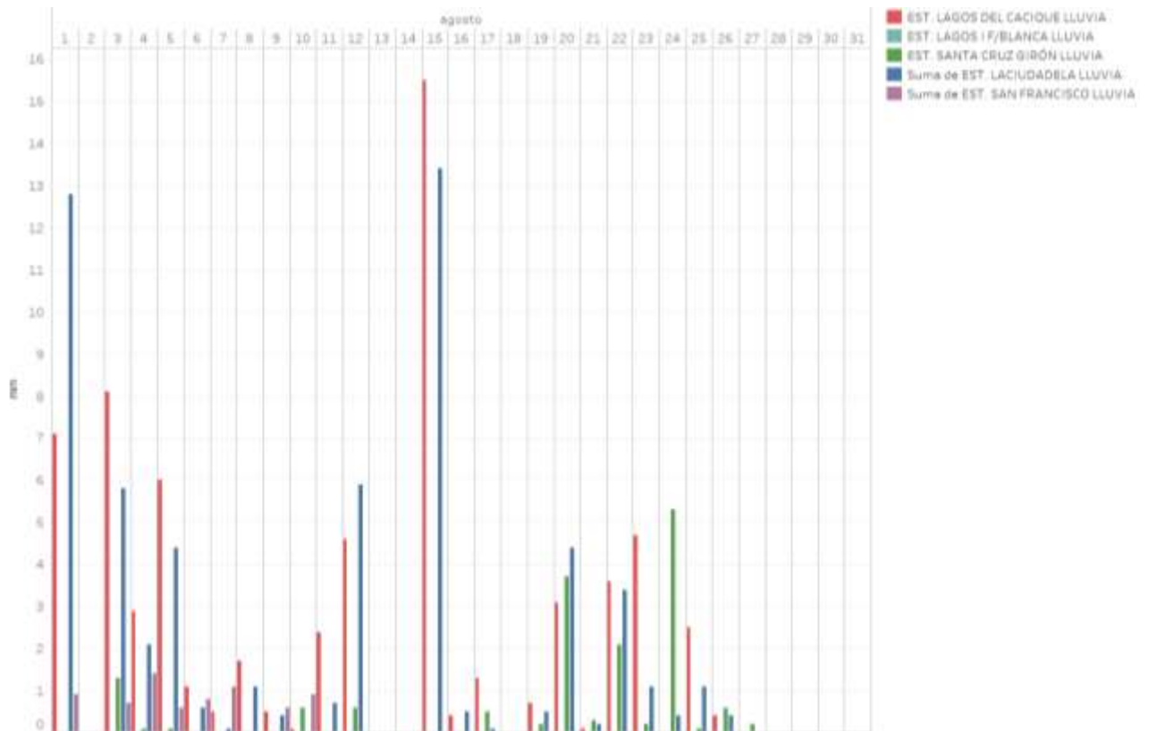
Figura 13 Variación diaria de la precipitación agosto 2020
