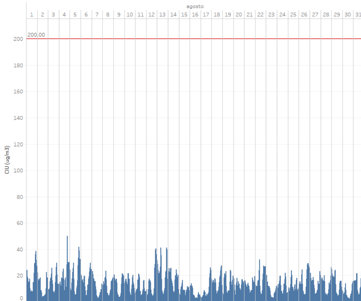
Figura 8 Comportamiento de las concentraciones 8h de NO 2 para agosto 2020 y comparación con Res 2254 de 2017
