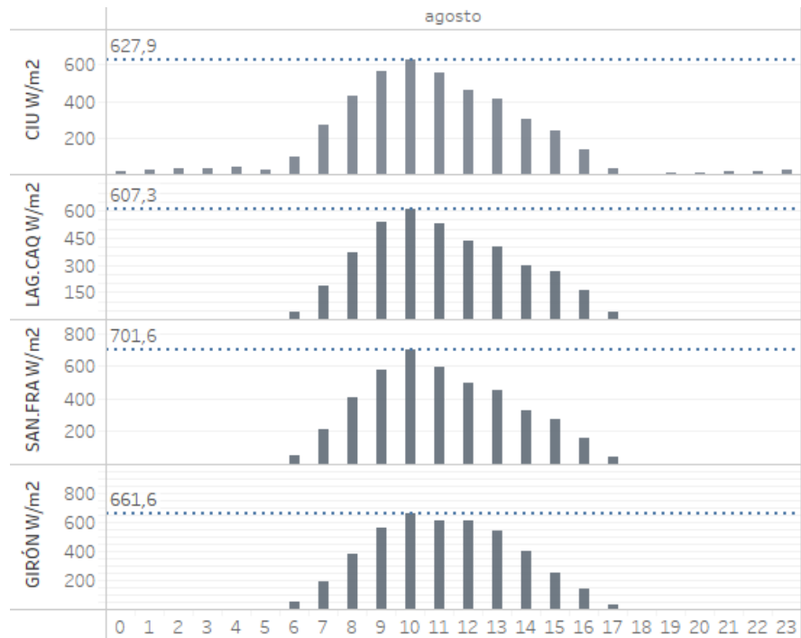
Figura 12 Comportamiento horario de la Radiación Solar entrante ( W/m^2 ) agosto
