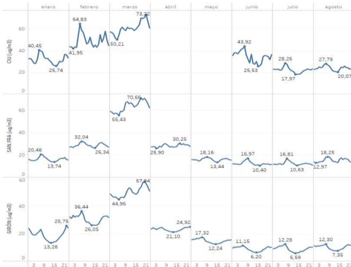
Figura 6 Comportamiento ciclo horario PM 2.5
