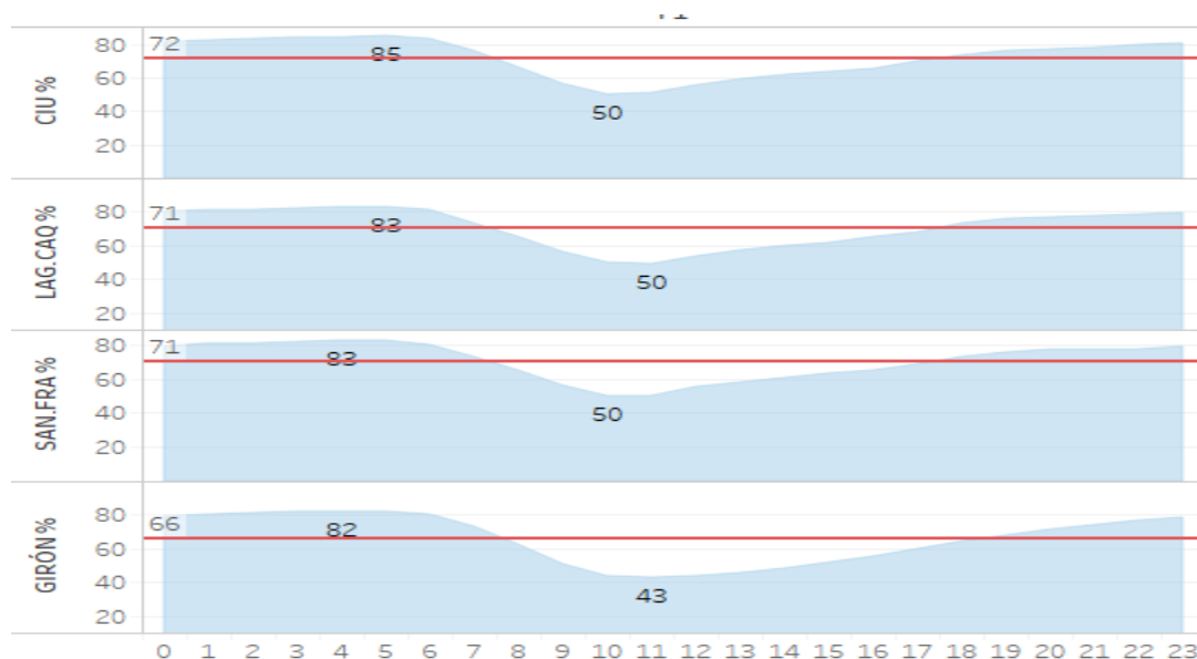
Figura 11 Comportamiento horario %Humedad Relativa
