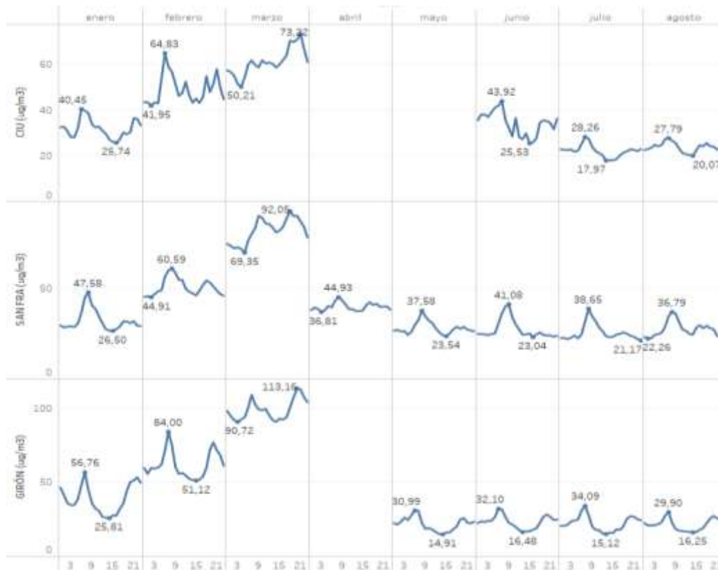
Figura 3 Comportamiento ciclo horario PM 10
