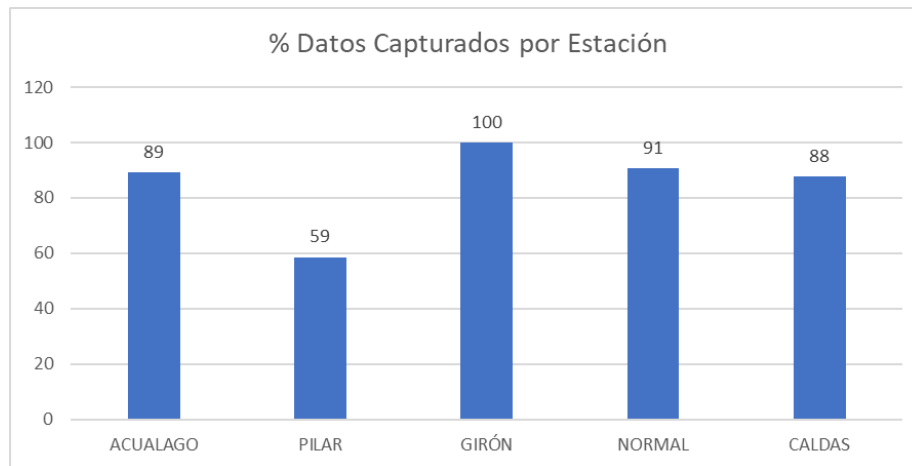
Figura 1 Porcentaje de Datos Válidos por ESTACIÓN
