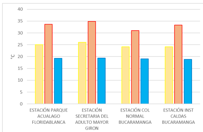
Figura 9 Resumen Temperaturas medias, máximas y mínima absolutas por estaciones y promedio área metropolitana agosto 2019.
