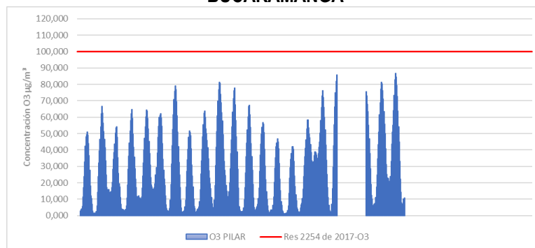
Figura 6 Comportamiento de las concentraciones 8h de O 3 para agosto 2019 y comparación con norma nacional.
