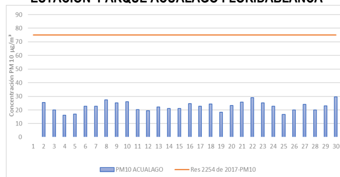
Figura 4 Comportamiento de las concentraciones diarias PM 10 para agosto de 2019
