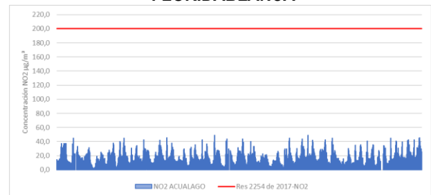
Figura 7 Comportamiento de las concentraciones 1h de NO 2 para agosto 2019
