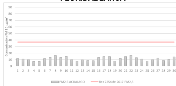
Figura 5 Comportamiento de las concentraciones diarias PM2.5 para agosto de 2019
