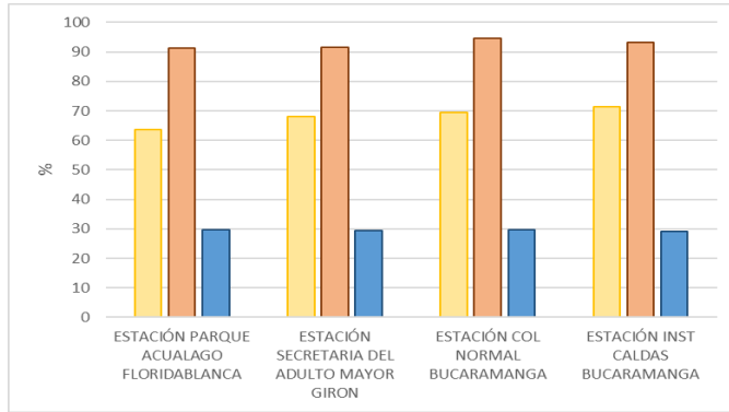
Figura 10 Resumen Humedad Relativa medias, máximas y mínima absolutas por estaciones y promedio área metropolitana agosto 2019.
