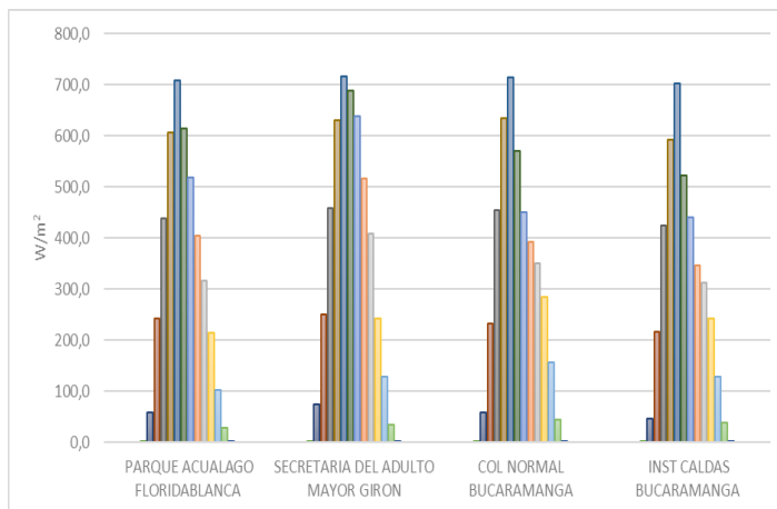
Figura 11 Comportamiento Horario Radiación Solar
