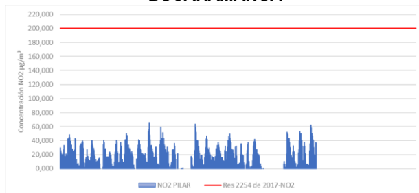
Figura 7 Comportamiento de las concentraciones 1h de NO 2 para agosto 2019
