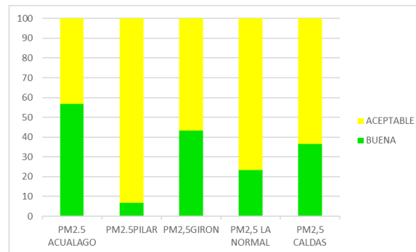
Figura 8 ICA por estación para PM2.5 para agosto
