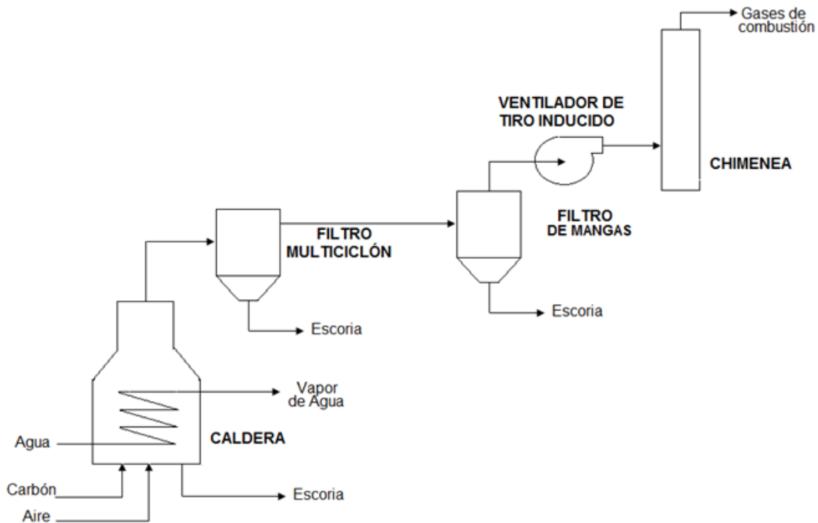
Ilustración 3. Diagrama de flujo del proceso asociado a la fuente CALDERA DISTRAL 200 BHP
