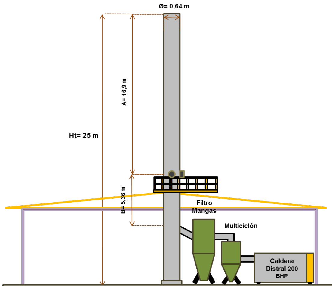
Ilustración 4. Diagrama del ducto CALDERA DISTRAL 200 BHP
